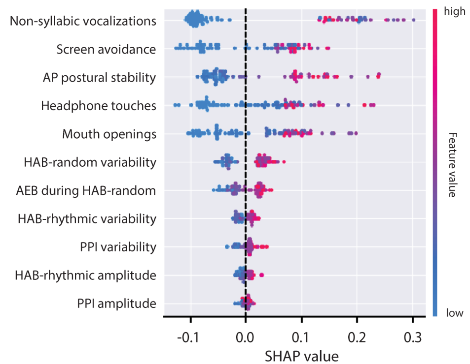
SHAP values
