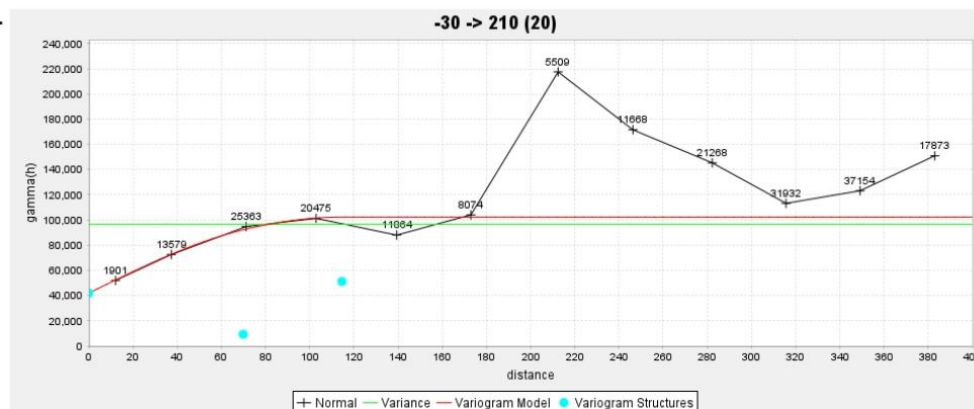
Mo
