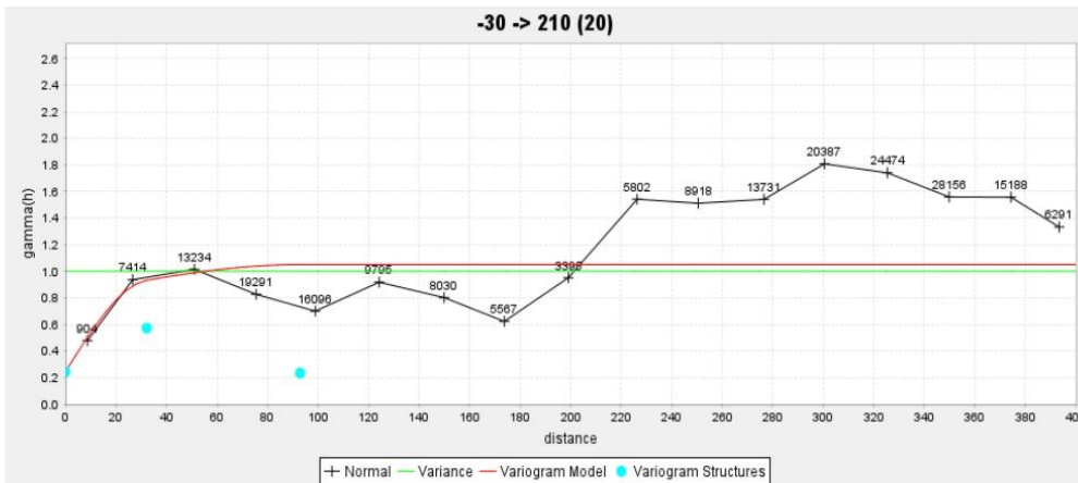
Nb
