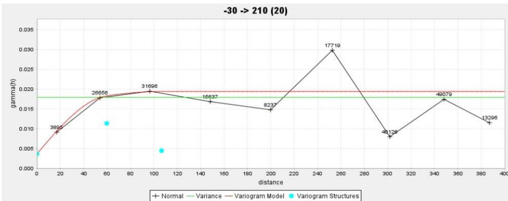
Mo
